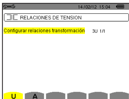
Figura 27: La pantalla Ratios de tensión en el menú Sensor y ratios en el caso de un montaje sin neutro
