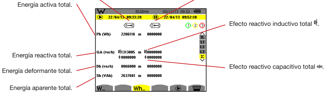
Figura 104: La pantalla de visualización de las energías consumidas y aportadas totales en \Sigma
