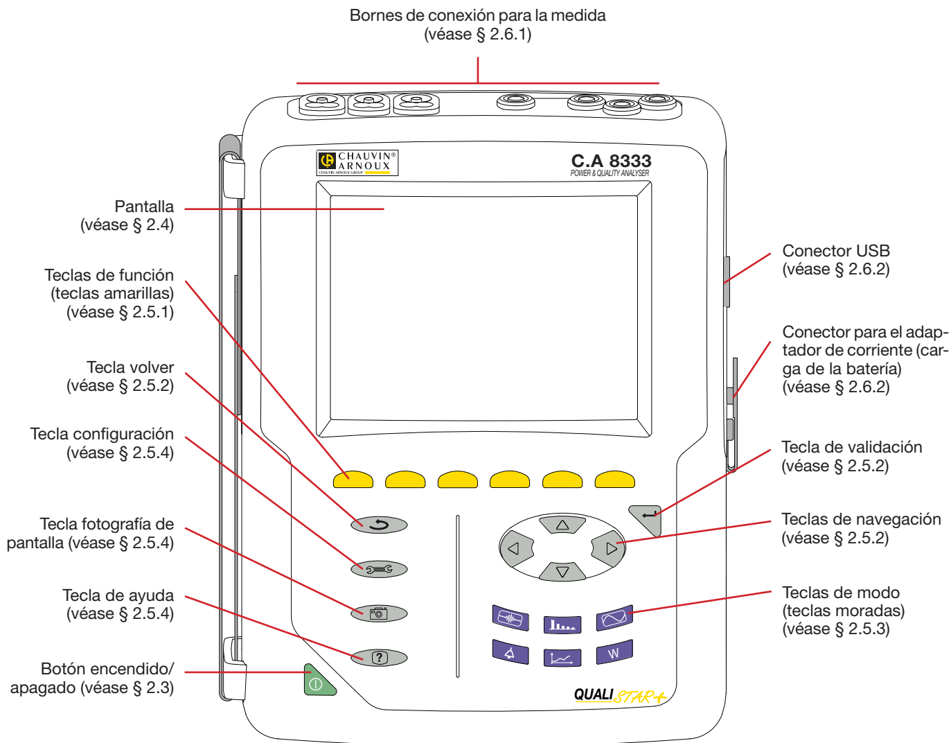
Figura 2: Vista general del Qualistar+
