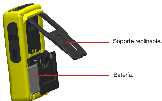
Figura 6: Soporte y tapa de acceso a la batería
