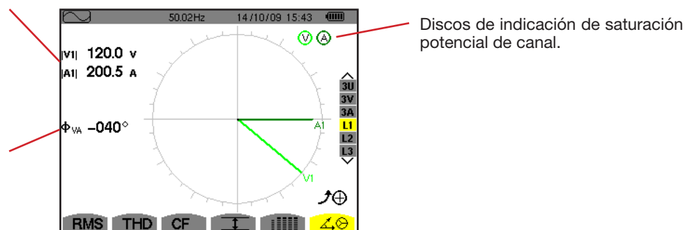
Figura 72: La pantalla de visualización del diagrama de Fresnel en L1
