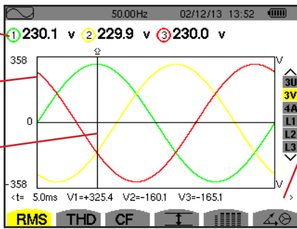
Figura 54: La pantalla de visualización RMS en 3V
