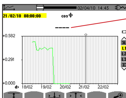
Figura 94: \cos \Phi (L1) para prematuro de la carga/cálculo de los valores
