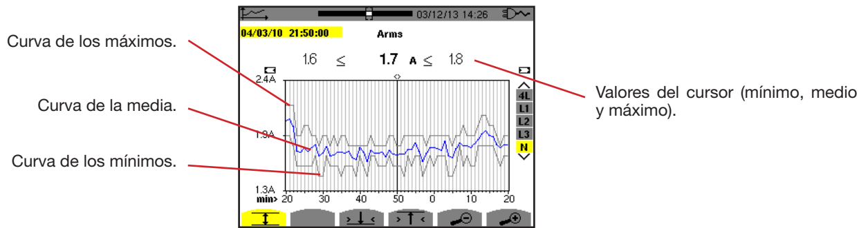
Figura 82: Arms (N) con MIN-AVG-MAX
